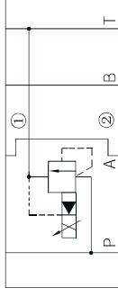
Model ZDBE6VP...
