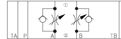
Model Z2FS10-...-3XJ/...(meter-out control)
